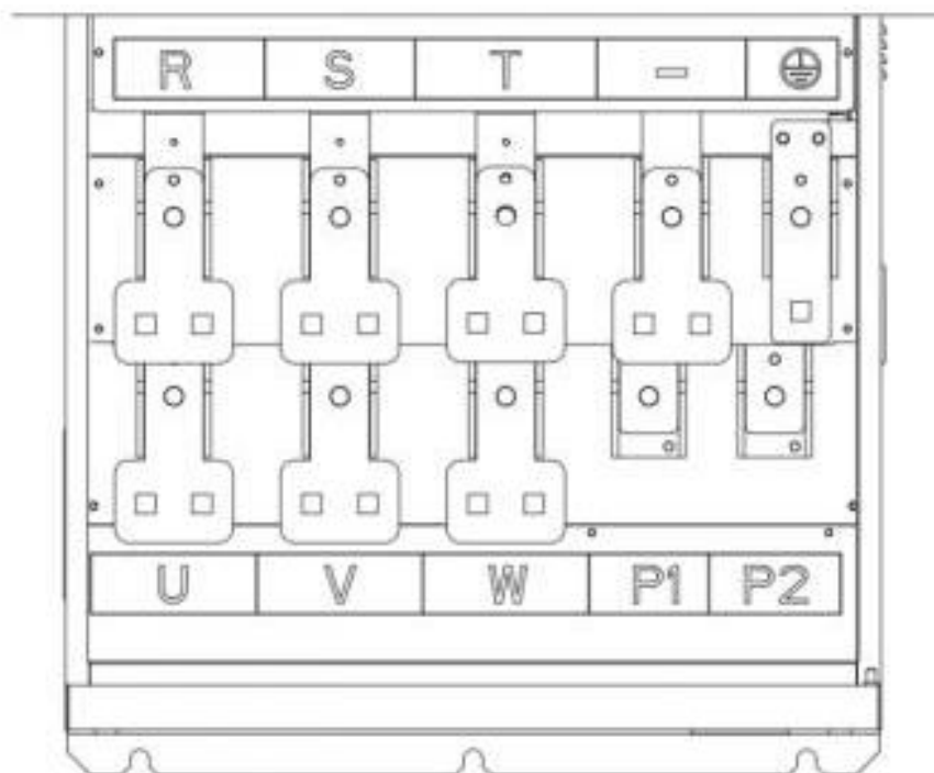
Рисунок 3 – Вид силовых клемм для VFD500-400G/450PT4
