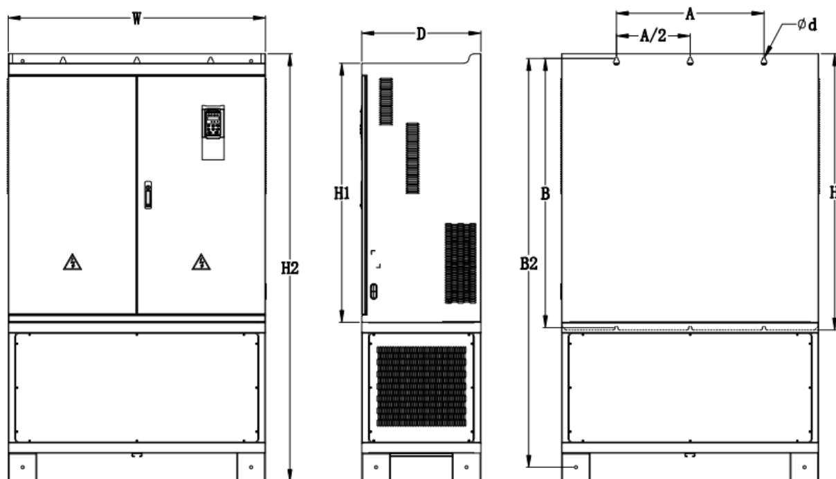
Рисунок 1 – габариты VFD500-400G/450PT4.
