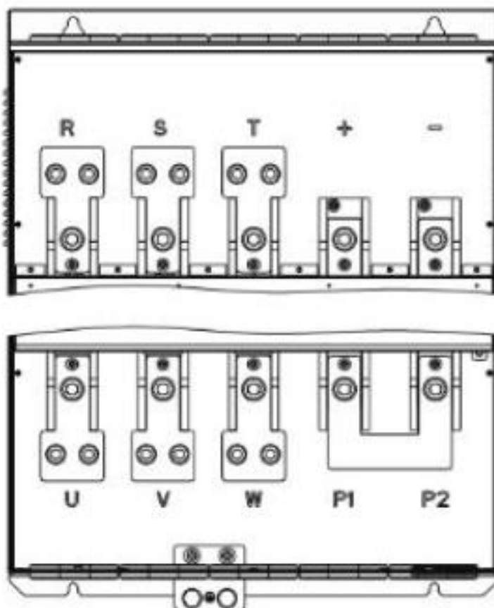
Рисунок 3 – Вид силовых клемм для VFD500-185G/200PT4
