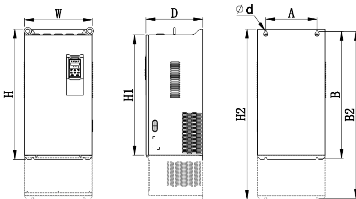
Рисунок 1 – габариты VFD500-185G/200PT4.
